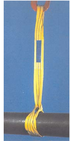
Båndstropp med vridde lærkledde øyer Sikkerhetsfaktor 7:1
